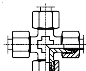
Cruzeta Igual Tubo - CI... Pag. 35
