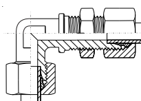
Joelho Tubo Comprido - JC... Pag. 38
