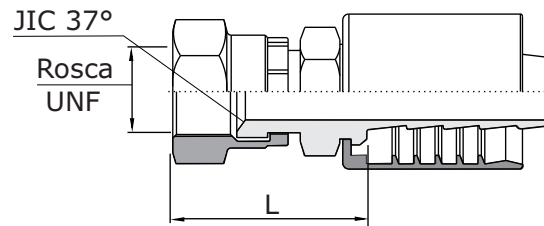
Femea Giratória JIC 37° (Female JIC 37° - Swivel)
