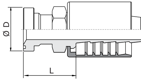
Flange SAE Código 61 Reto - 3000 PSI (SAE Code 61 Flange Head)
