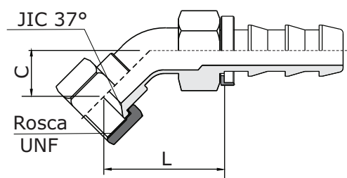
Femea Giratória JIC 37° Curva 45° (Female JIC 37° - Swivel - 45° Elbow)
